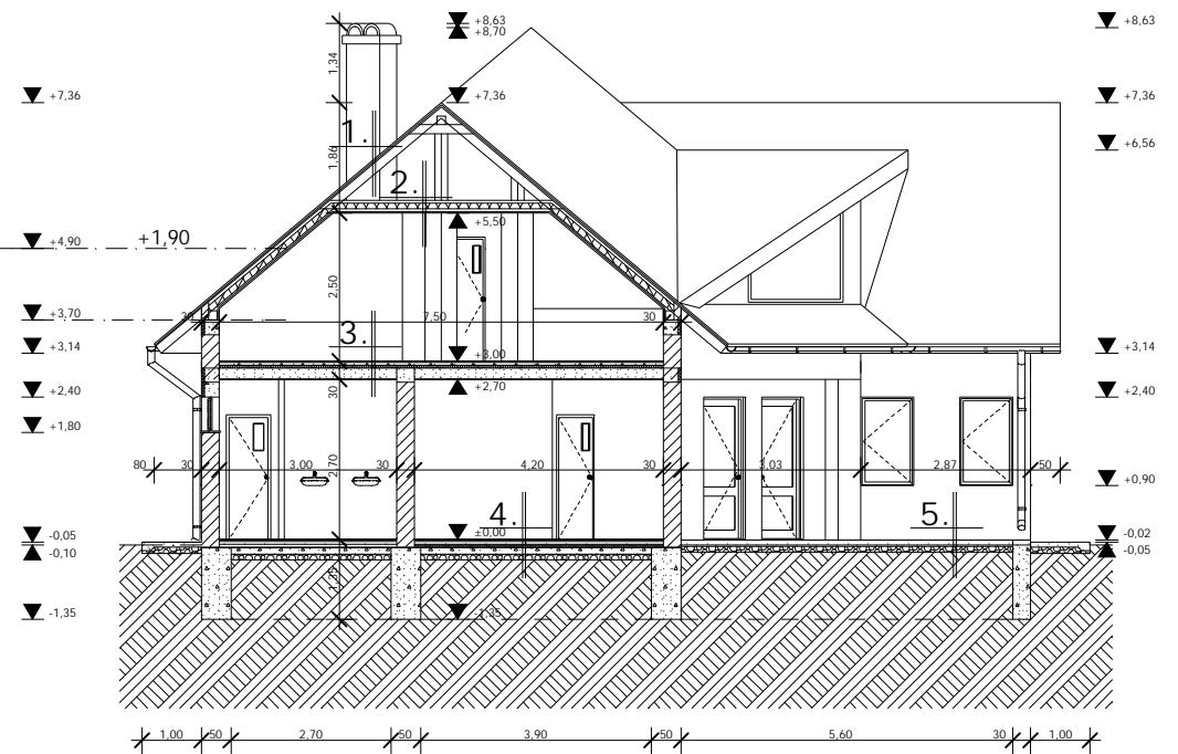
B-B METSZET M=1:100
