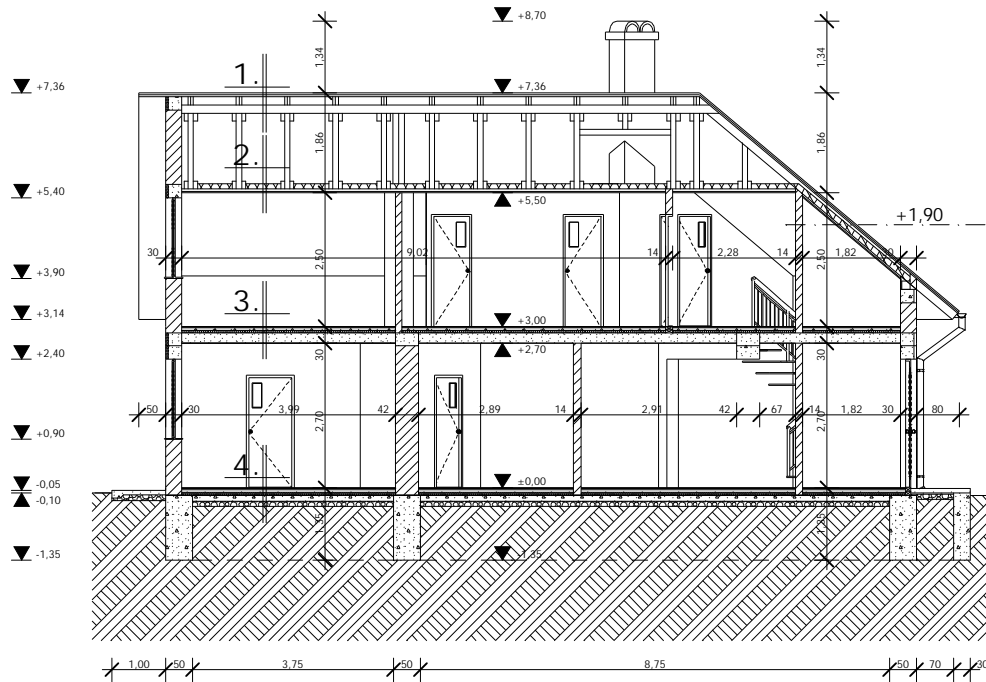
A-A METSZET M=1:100
